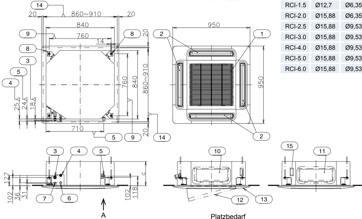
Platzbedarf
