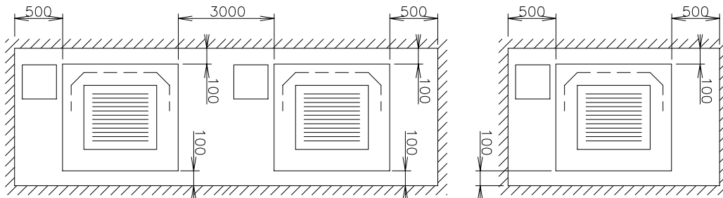
Platzbedarf
