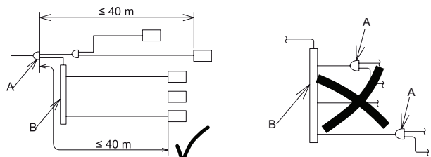
A Leitungsabzweigung B Verteiler (Kopfabzweigung)
