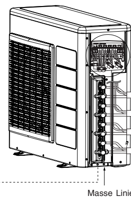
Nach Entfernen der Abdeckung, Verbindungskabel anschließen und mit Schrauben befestigen.
