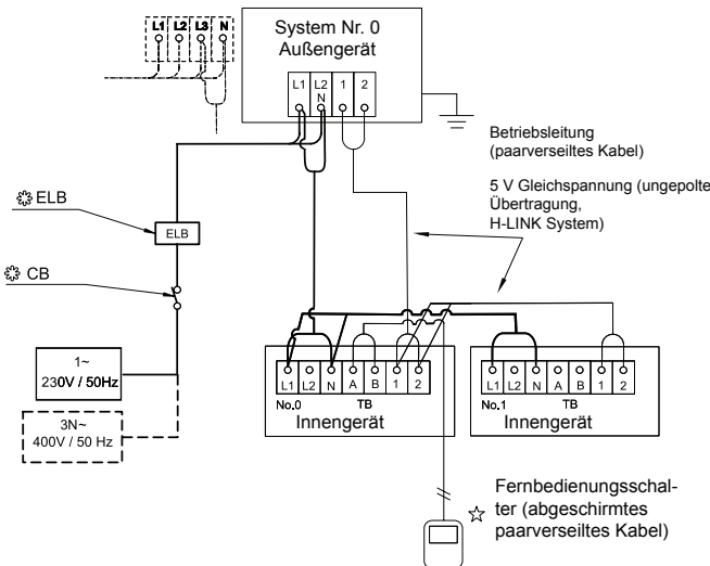
Stromversorgung vom Außengerät IVX zum Innengerät (Beispiel)
