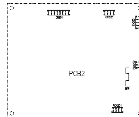
For RPI-(2.5-6.0)FSN4E
