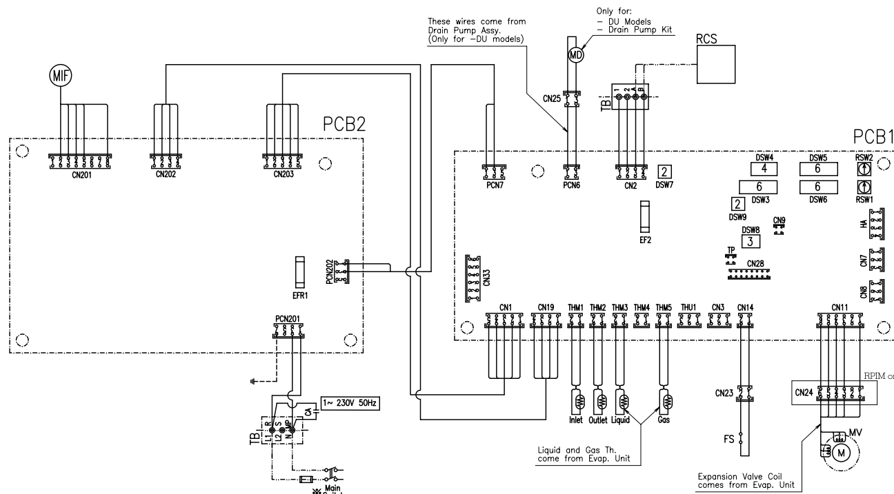
For RPI-(2.5-6.0)FSN4E
